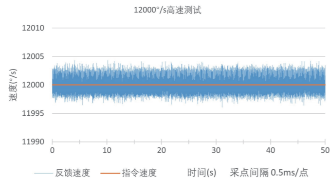
Theta轴空载转速12000°/s (2000rpm) 下高速运动的速度反馈
